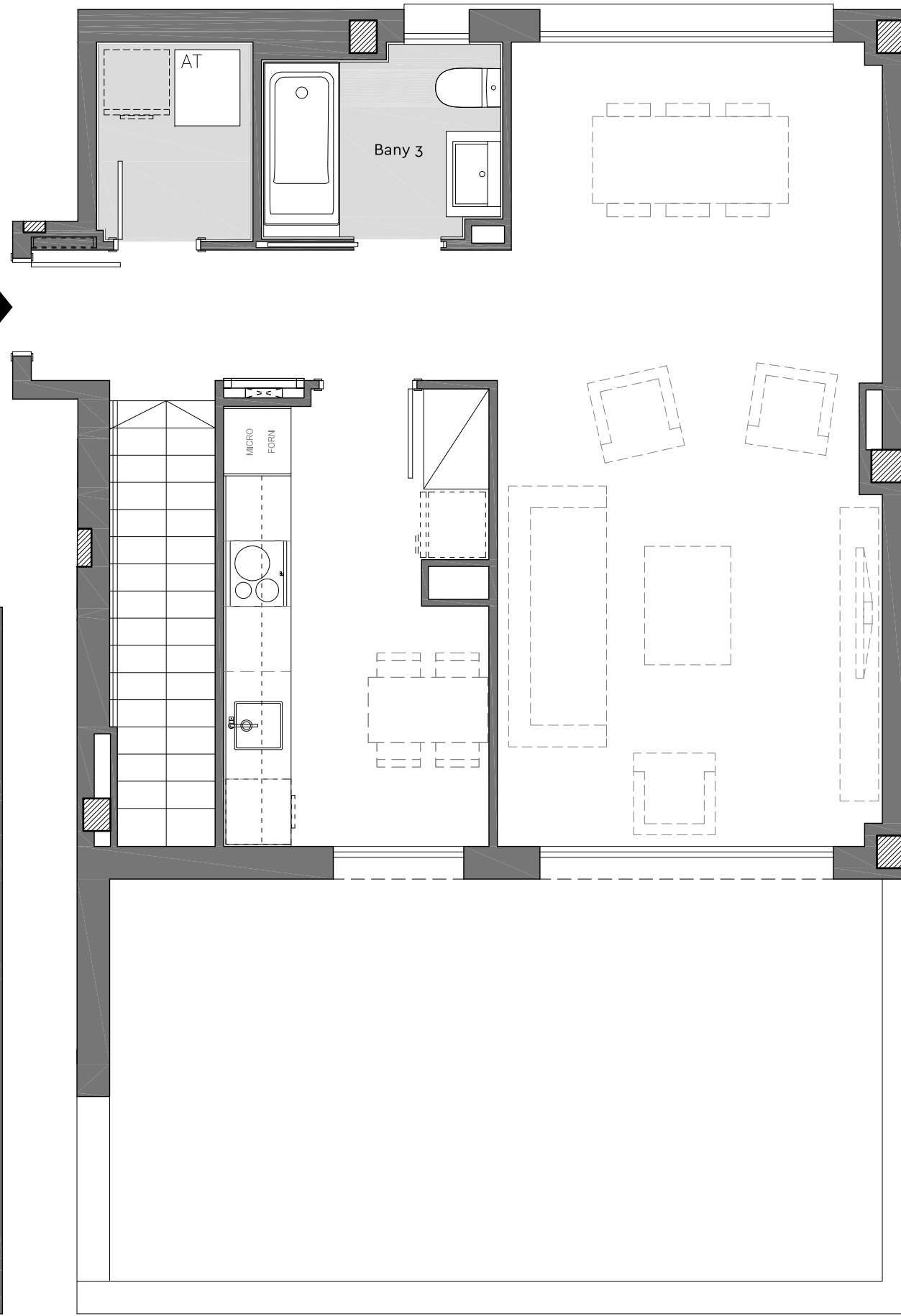
PLANTA SUPERIOR
